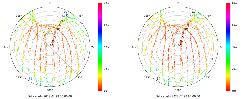
Skyplot for station IZAN. Parameter M1C Data file IZAN00ESP_R_2022204.xtr Skyplot for station IZAN. Parameter M2C Data file IZAN00ESP_R_2022204.xtr
