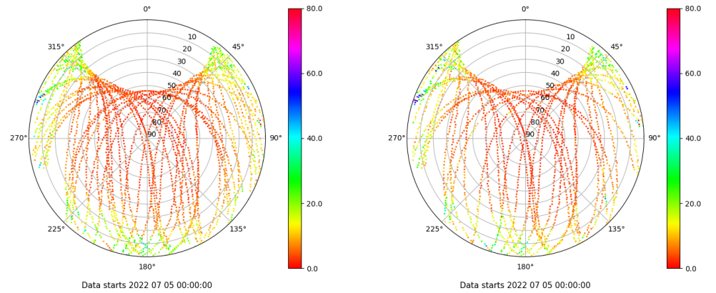
Skyplot for station IZAN. Parameter M1C Data file IZAN00ESP_R_2022186.xtr Skyplot for station IZAN. Parameter M2S Data file IZAN00ESP_R_2022186.xtr
