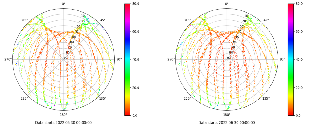
Skyplot for station IZAN. Parameter M1C Data file IZAN00ESP_R_2022181.xtr Skyplot for station IZAN. Parameter M2C Data file IZAN00ESP_R_2022181.xtr
