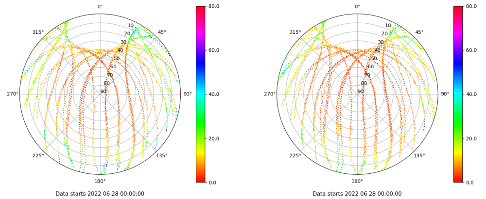
Skyplot for station IZAN. Parameter M1C Data file IZAN00ESP_R_2022179.xtr Skyplot for station IZAN. Parameter M2C Data file IZAN00ESP_R_2022179.xtr
