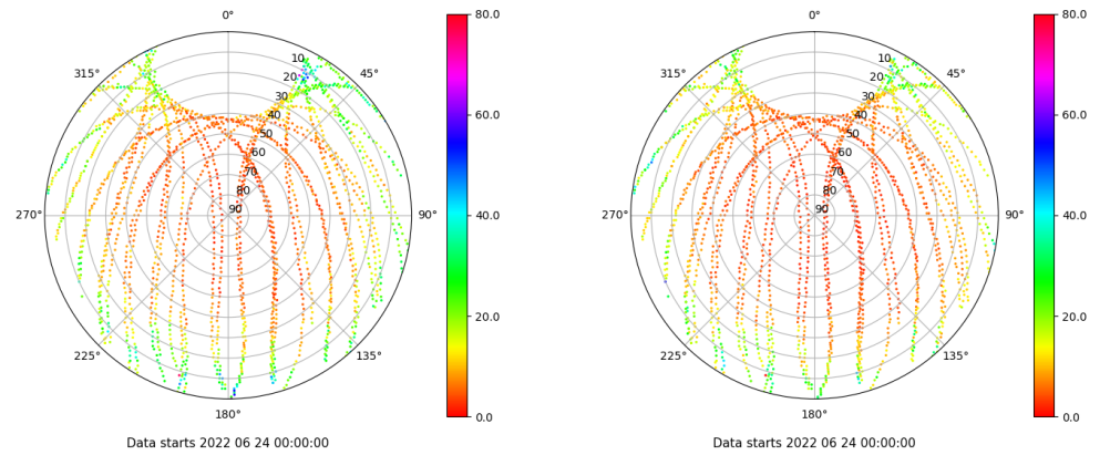
Skyplot for station IZAN. Parameter M1C Data file IZAN00ESP_R_2022175.xtr Skyplot for station IZAN. Parameter M2C Data file IZAN00ESP_R_2022175.xtr
