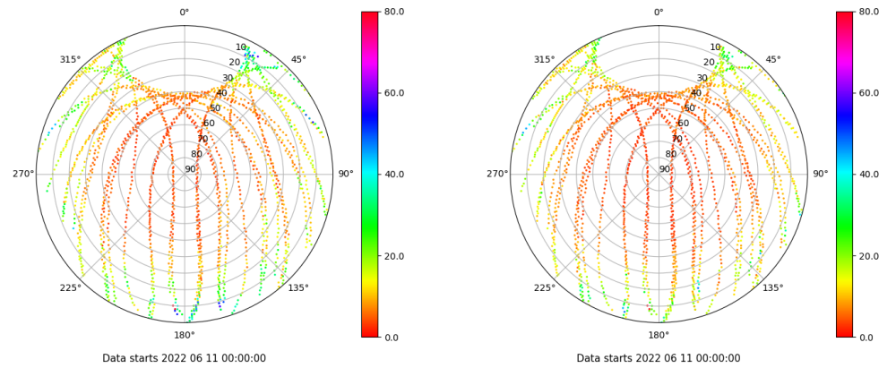
Skyplot for station IZAN. Parameter M1C Data file IZAN00ESP_R_2022162.xtr Skyplot for station IZAN. Parameter M2C Data file IZAN00ESP_R_2022162.xtr
