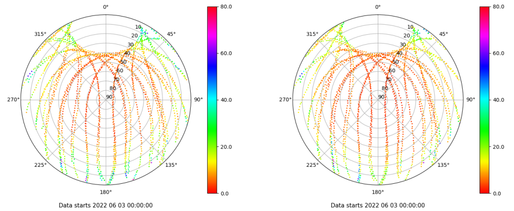
Skyplot for station IZAN. Parameter M1C Data file IZAN00ESP_R_2022154.xtr Skyplot for station IZAN. Parameter M2C Data file IZAN00ESP_R_2022154.xtr
