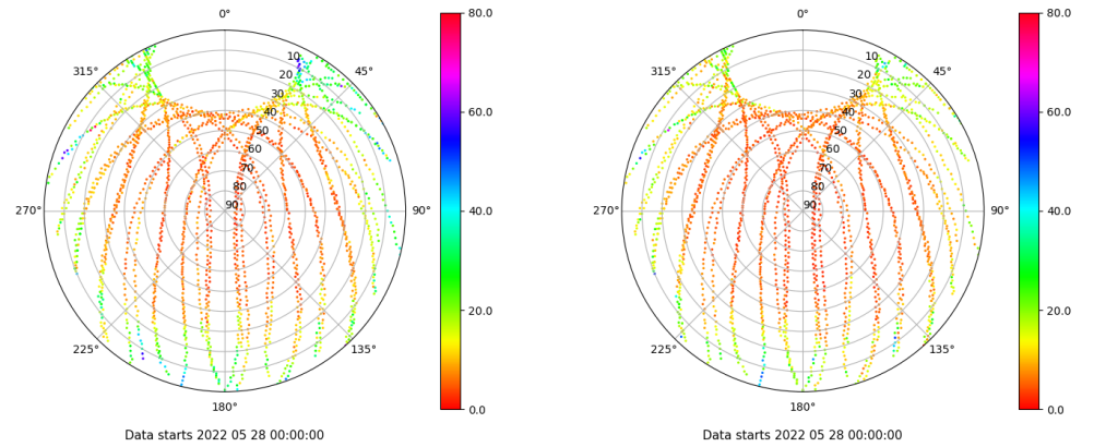
Skyplot for station IZAN. Parameter M1C Data file IZAN00ESP_R_2022148.xtr Skyplot for station IZAN. Parameter M2C Data file IZAN00ESP_R_2022148.xtr
