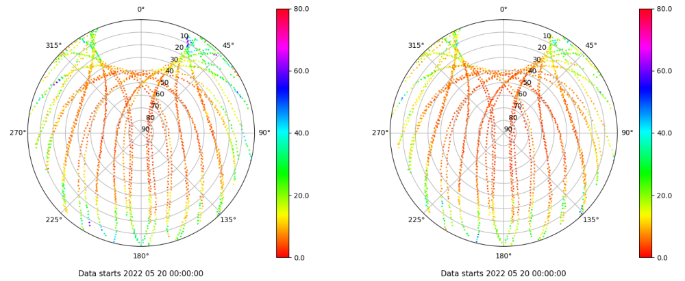
Skyplot for station IZAN. Parameter M1C Data file IZAN00ESP_R_2022140.xtr Skyplot for station IZAN. Parameter M2C Data file IZAN00ESP_R_2022140.xtr
