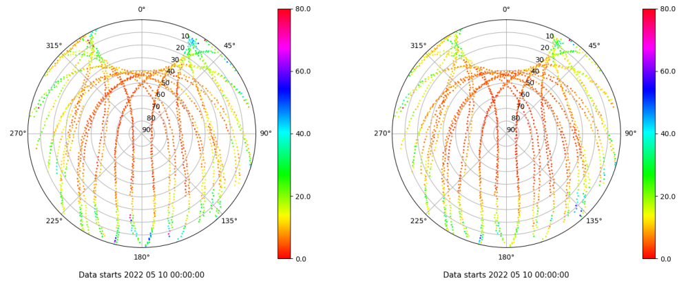
Skyplot for station IZAN. Parameter M1C Data file IZAN00ESP_R_2022130.xtr Skyplot for station IZAN. Parameter M2C Data file IZAN00ESP_R_2022130.xtr
