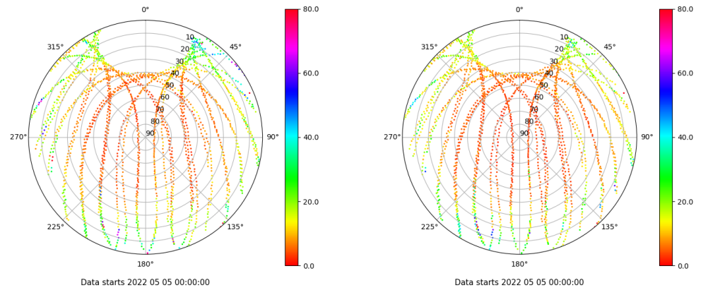
Skyplot for station IZAN. Parameter M1C Data file IZAN00ESP_R_2022125.xtr Skyplot for station IZAN. Parameter M2C Data file IZAN00ESP_R_2022125.xtr
