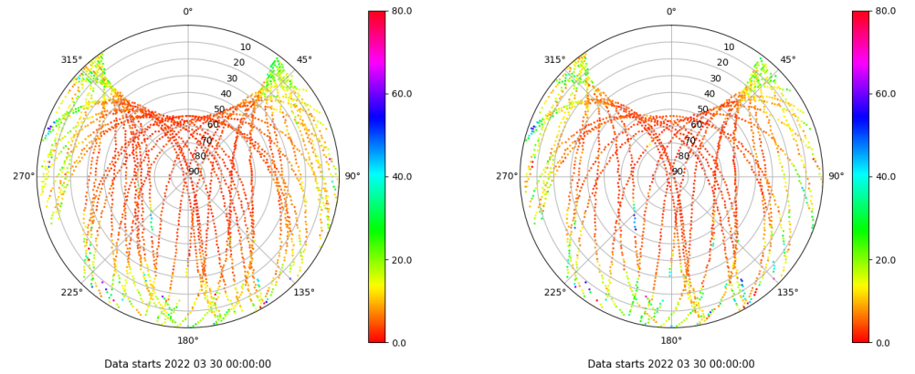
Skyplot for station IZAN. Parameter M1C Data file IZAN00ESP_R_2022089.xtr Skyplot for station IZAN. Parameter M2S Data file IZAN00ESP_R_2022089.xtr
