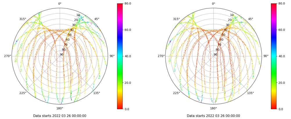
Skyplot for station IZAN. Parameter M1C Data file IZAN00ESP_R_2022085.xtr Skyplot for station IZAN. Parameter M2C Data file IZAN00ESP_R_2022085.xtr
