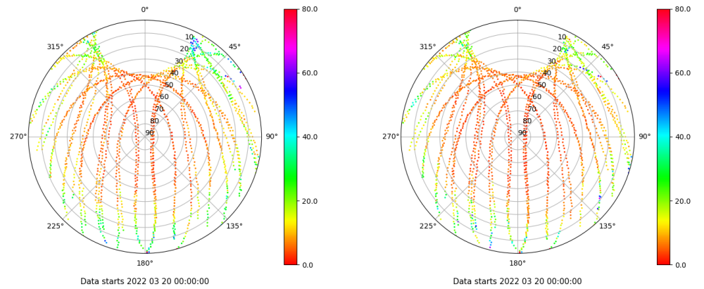
Skyplot for station IZAN. Parameter M1C Data file IZAN00ESP_R_2022079.xtr Skyplot for station IZAN. Parameter M2C Data file IZAN00ESP_R_2022079.xtr
