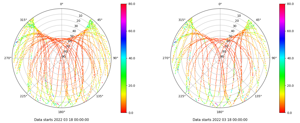
Skyplot for station IZAN. Parameter M1C Data file IZAN00ESP_R_2022077.xtr Skyplot for station IZAN. Parameter M2S Data file IZAN00ESP_R_2022077.xtr
