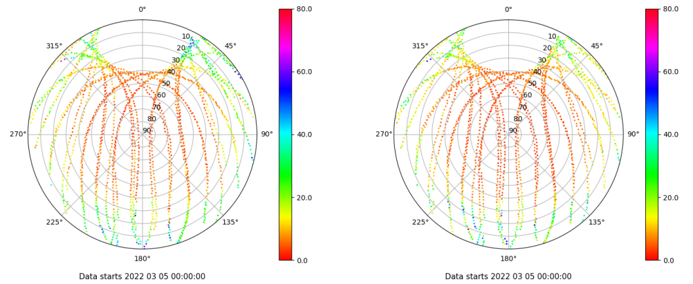
Skyplot for station IZAN. Parameter M1C Data file IZAN00ESP_R_2022064.xtr Skyplot for station IZAN. Parameter M2C Data file IZAN00ESP_R_2022064.xtr
