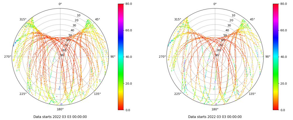
Skyplot for station IZAN. Parameter M1C Data file IZAN00ESP_R_2022062.xtr Skyplot for station IZAN. Parameter M2S Data file IZAN00ESP_R_2022062.xtr
