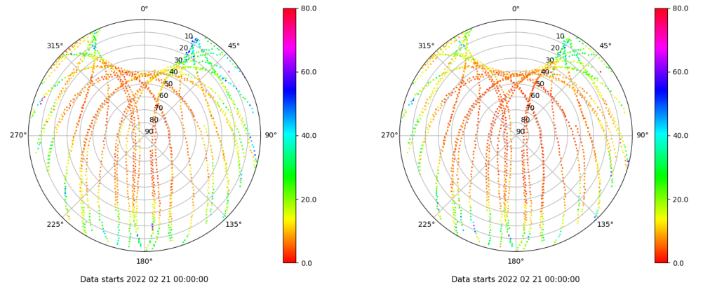
Skyplot for station IZAN. Parameter M1C Data file IZAN00ESP_R_2022052.xtr Skyplot for station IZAN. Parameter M2C Data file IZAN00ESP_R_2022052.xtr
