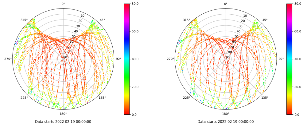
Skyplot for station IZAN. Parameter M1C Data file IZAN00ESP_R_2022050.xtr Skyplot for station IZAN. Parameter M2S Data file IZAN00ESP_R_2022050.xtr
