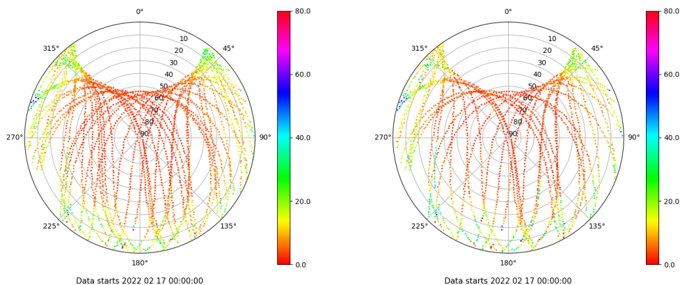
Skyplot for station IZAN. Parameter M1C Data file IZAN00ESP_R_2022048.xtr Skyplot for station IZAN. Parameter M2S Data file IZAN00ESP_R_2022048.xtr
