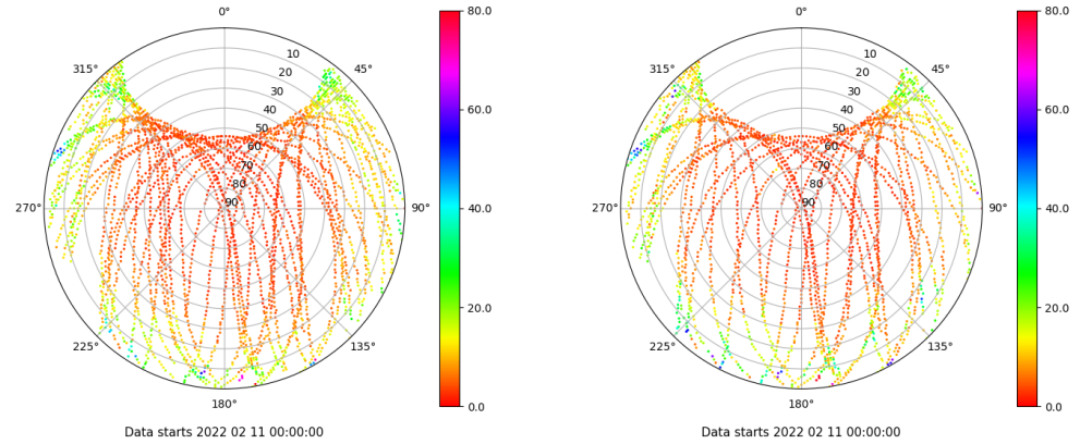
Skyplot for station IZAN. Parameter M1C Data file IZAN00ESP_R_2022042.xtr Skyplot for station IZAN. Parameter M2S Data file IZAN00ESP_R_2022042.xtr
