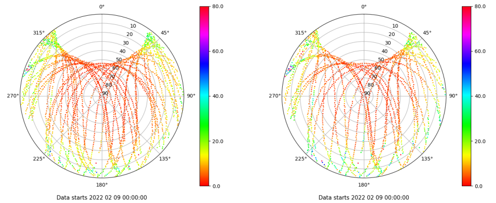
Skyplot for station IZAN. Parameter M1C Data file IZAN00ESP_R_2022040.xtr Skyplot for station IZAN. Parameter M2S Data file IZAN00ESP_R_2022040.xtr
