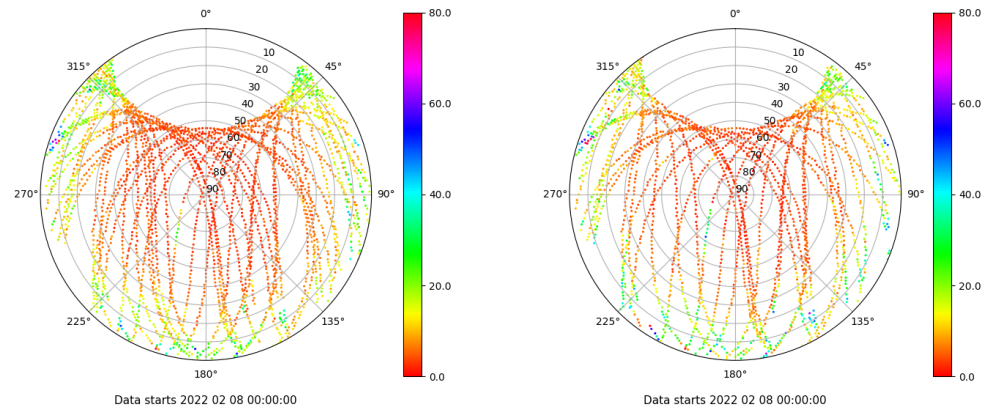
Skyplot for station IZAN. Parameter M1C Data file IZAN00ESP_R_2022039.xtr Skyplot for station IZAN. Parameter M2S Data file IZAN00ESP_R_2022039.xtr
