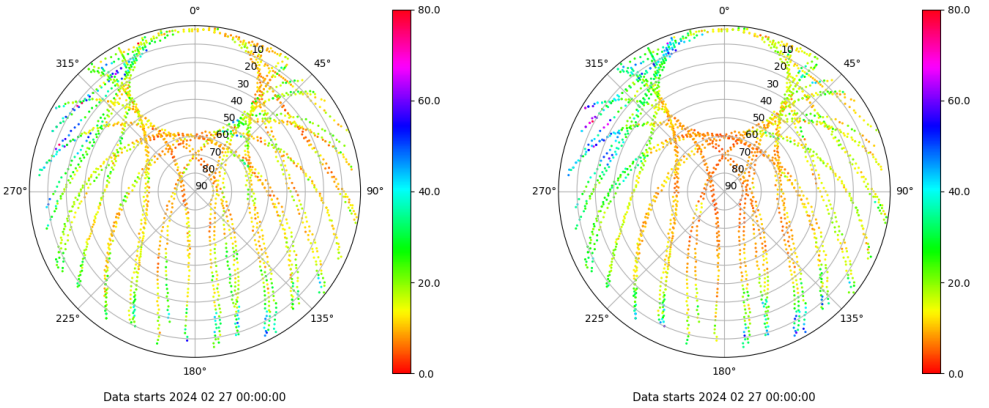
Skyplot for station GIRO. Parameter M1C Data file GIRO00ESP_R_2024058.xtr Skyplot for station GIRO. Parameter M2P Data file GIRO00ESP_R_2024058.xtr
