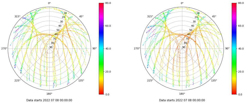
Skyplot for station GIRO. Parameter M1C Data file GIRO00ESP_R_2022189.xtr Skyplot for station GIRO. Parameter M2P Data file GIRO00ESP_R_2022189.xtr
