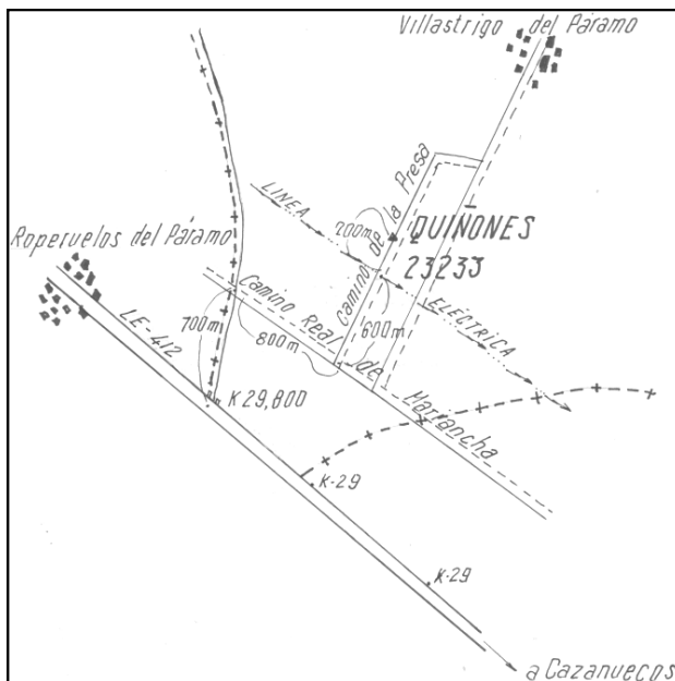
Quinones
