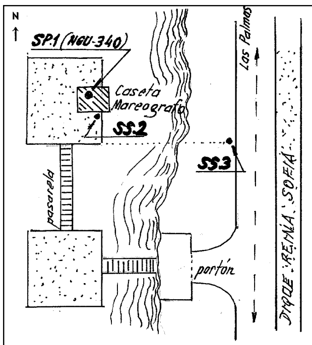
Gran Canaria NGU340 (Mareógrafo Dique Reina Sofía)
