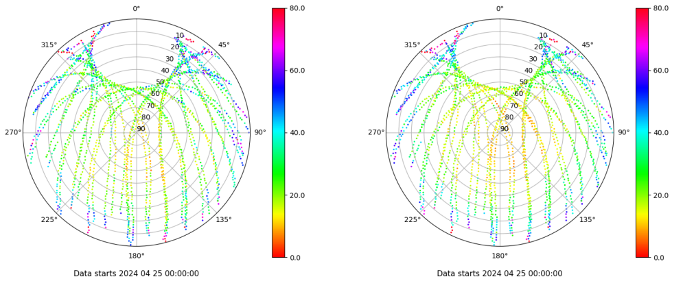
Skyplot for station ZFRA. Parameter M1C Data file ZFRA00ESP_R_2024116.xtr Skyplot for station ZFRA. Parameter M2P Data file ZFRA00ESP_R_2024116.xtr
