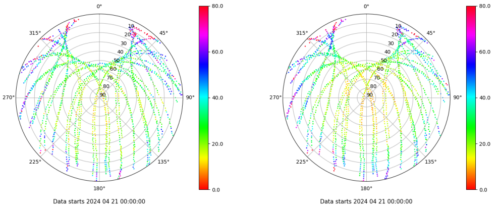
Skyplot for station ZFRA. Parameter M1C Data file ZFRA00ESP_R_2024112.xtr Skyplot for station ZFRA. Parameter M2P Data file ZFRA00ESP_R_2024112.xtr
