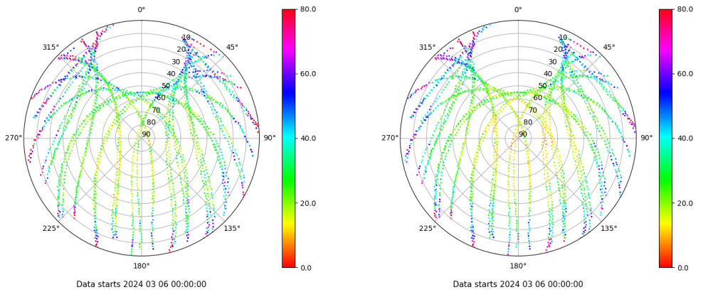
Skyplot for station ZFRA. Parameter M1C Data file ZFRA00ESP_R_2024066.xtr Skyplot for station ZFRA. Parameter M2P Data file ZFRA00ESP_R_2024066.xtr
