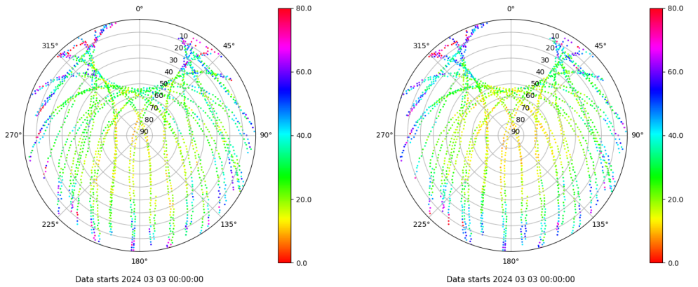
Skyplot for station ZFRA. Parameter M1C Data file ZFRA00ESP_R_2024063.xtr Skyplot for station ZFRA. Parameter M2P Data file ZFRA00ESP_R_2024063.xtr
