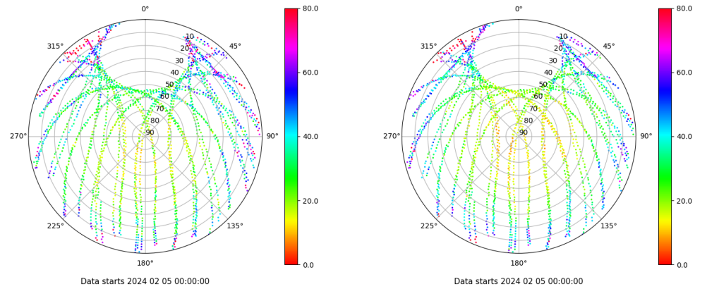
Skyplot for station ZFRA. Parameter M1C Data file ZFRA00ESP_R_2024036.xtr Skyplot for station ZFRA. Parameter M2P Data file ZFRA00ESP_R_2024036.xtr
