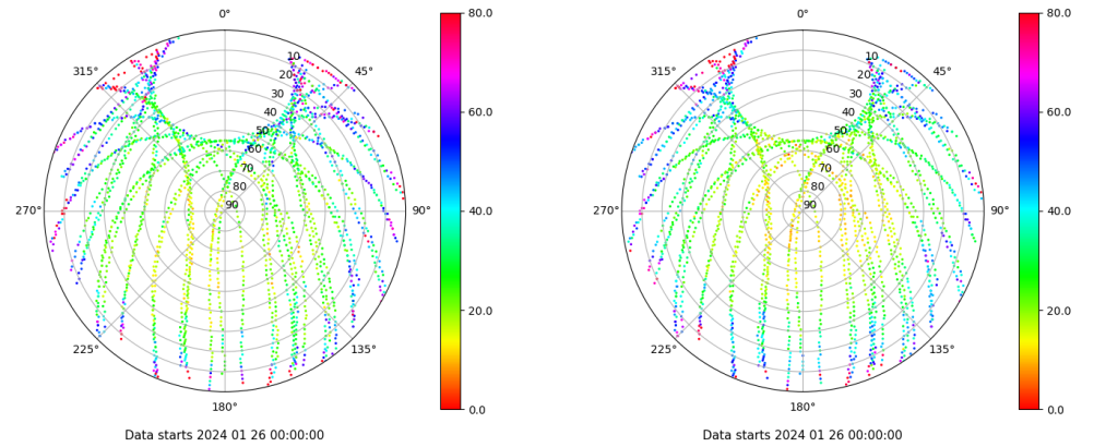
Skyplot for station ZFRA. Parameter M1C Data file ZFRA00ESP_R_2024026.xtr Skyplot for station ZFRA. Parameter M2P Data file ZFRA00ESP_R_2024026.xtr
