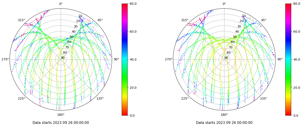
Skyplot for station ZFRA. Parameter M1C Data file ZFRA00ESP_R_2023269.xtr Skyplot for station ZFRA. Parameter M2P Data file ZFRA00ESP_R_2023269.xtr
