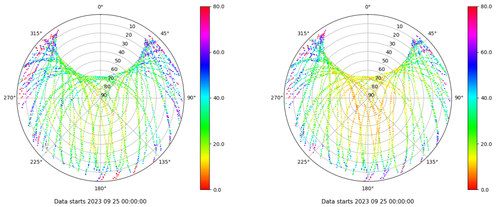
Skyplot for station ZFRA. Parameter M1C Data file ZFRA00ESP_R_2023268.xtr Skyplot for station ZFRA. Parameter M2W Data file ZFRA00ESP_R_2023268.xtr
