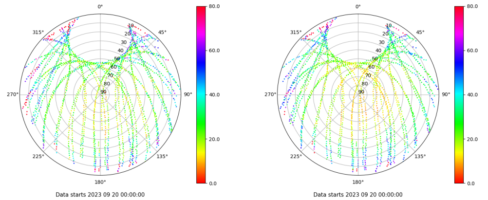
Skyplot for station ZFRA. Parameter M1C Data file ZFRA00ESP_R_2023263.xtr Skyplot for station ZFRA. Parameter M2P Data file ZFRA00ESP_R_2023263.xtr
