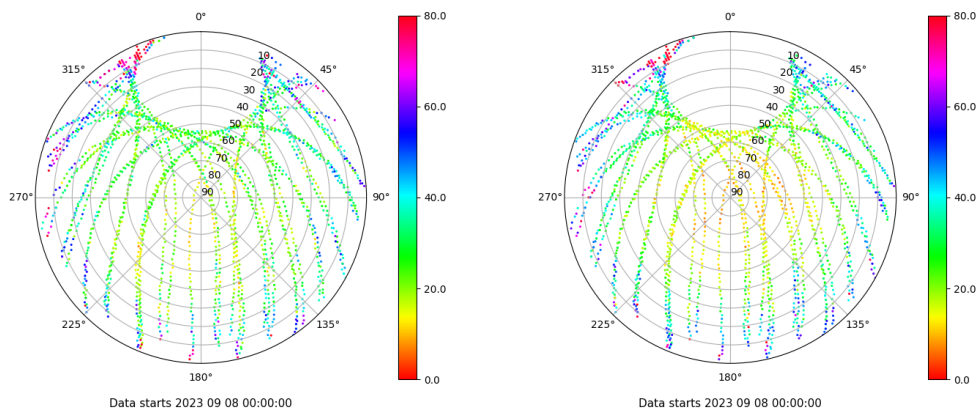
Skyplot for station ZFRA. Parameter M1C Data file ZFRA00ESP_R_2023251.xtr Skyplot for station ZFRA. Parameter M2P Data file ZFRA00ESP_R_2023251.xtr
