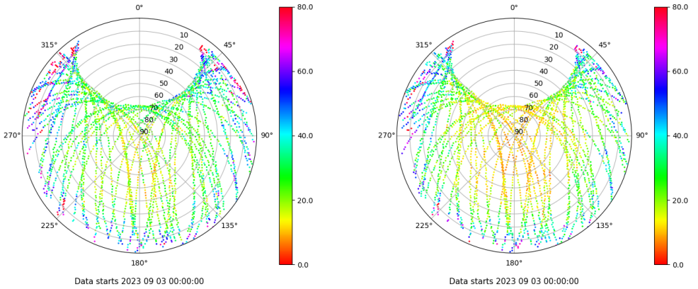
Skyplot for station ZFRA. Parameter M1C Data file ZFRA00ESP_R_2023246.xtr Skyplot for station ZFRA. Parameter M2W Data file ZFRA00ESP_R_2023246.xtr
