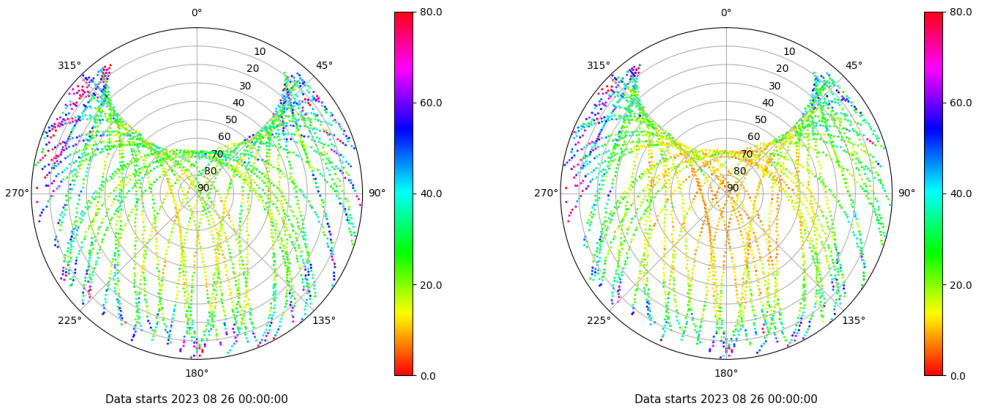
Skyplot for station ZFRA. Parameter M1C Data file ZFRA00ESP_R_2023238.xtr Skyplot for station ZFRA. Parameter M2W Data file ZFRA00ESP_R_2023238.xtr
