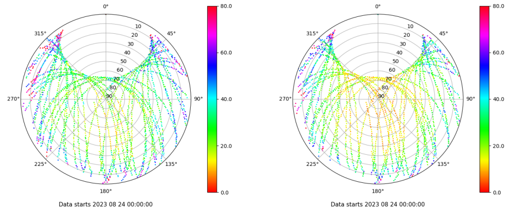
Skyplot for station ZFRA. Parameter M1C Data file ZFRA00ESP_R_2023236.xtr Skyplot for station ZFRA. Parameter M2W Data file ZFRA00ESP_R_2023236.xtr
