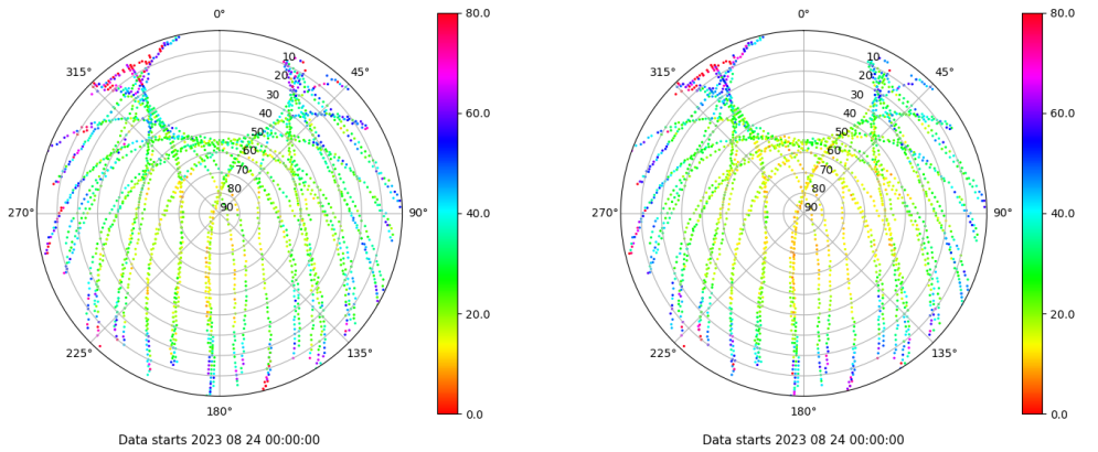
Skyplot for station ZFRA. Parameter M1C Data file ZFRA00ESP_R_2023236.xtr Skyplot for station ZFRA. Parameter M2P Data file ZFRA00ESP_R_2023236.xtr
