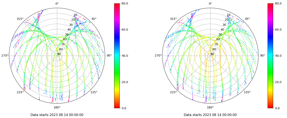
Skyplot for station ZFRA. Parameter M1C Data file ZFRA00ESP_R_2023226.xtr Skyplot for station ZFRA. Parameter M2P Data file ZFRA00ESP_R_2023226.xtr
