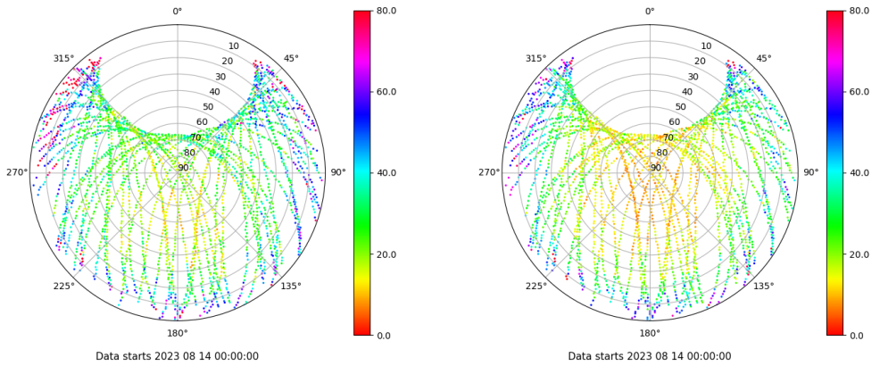
Skyplot for station ZFRA. Parameter M1C Data file ZFRA00ESP_R_2023226.xtr Skyplot for station ZFRA. Parameter M2W Data file ZFRA00ESP_R_2023226.xtr
