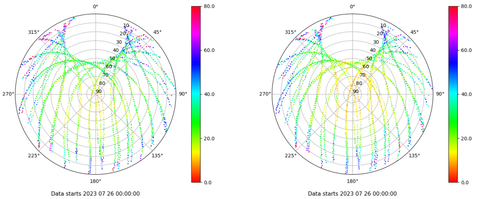
Skyplot for station ZFRA. Parameter M1C Data file ZFRA00ESP_R_2023207.xtr Skyplot for station ZFRA. Parameter M2P Data file ZFRA00ESP_R_2023207.xtr
