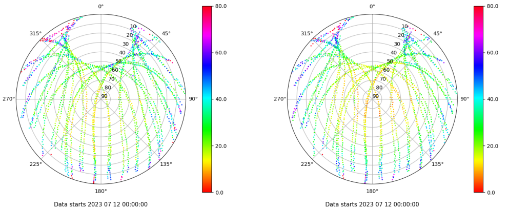
Skyplot for station ZFRA. Parameter M1C Data file ZFRA00ESP_R_2023193.xtr Skyplot for station ZFRA. Parameter M2P Data file ZFRA00ESP_R_2023193.xtr
