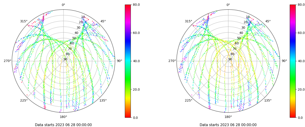
Skyplot for station ZFRA. Parameter M1C Data file ZFRA00ESP_R_2023179.xtr Skyplot for station ZFRA. Parameter M2P Data file ZFRA00ESP_R_2023179.xtr
