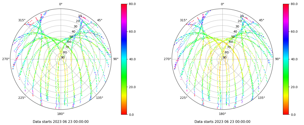
Skyplot for station ZFRA. Parameter M1C Data file ZFRA00ESP_R_2023174.xtr Skyplot for station ZFRA. Parameter M2P Data file ZFRA00ESP_R_2023174.xtr
