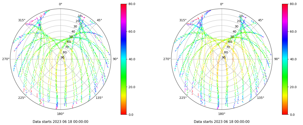
Skyplot for station ZFRA. Parameter M1C Data file ZFRA00ESP_R_2023169.xtr Skyplot for station ZFRA. Parameter M2P Data file ZFRA00ESP_R_2023169.xtr
