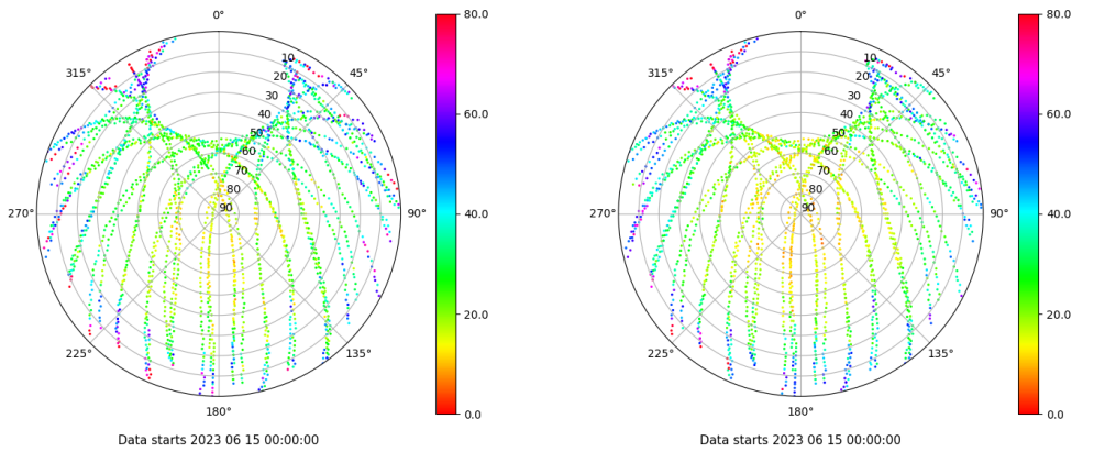
Skyplot for station ZFRA. Parameter M1C Data file ZFRA00ESP_R_2023166.xtr Skyplot for station ZFRA. Parameter M2P Data file ZFRA00ESP_R_2023166.xtr
