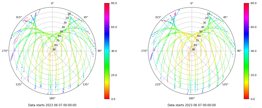
Skyplot for station ZFRA. Parameter M1C Data file ZFRA00ESP_R_2023158.xtr Skyplot for station ZFRA. Parameter M2P Data file ZFRA00ESP_R_2023158.xtr
