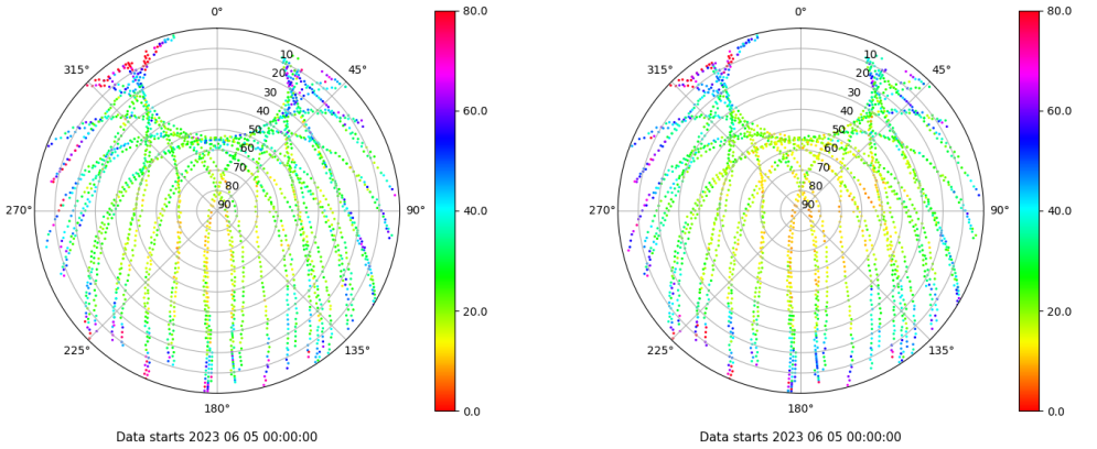
Skyplot for station ZFRA. Parameter M1C Data file ZFRA00ESP_R_2023156.xtr Skyplot for station ZFRA. Parameter M2P Data file ZFRA00ESP_R_2023156.xtr
