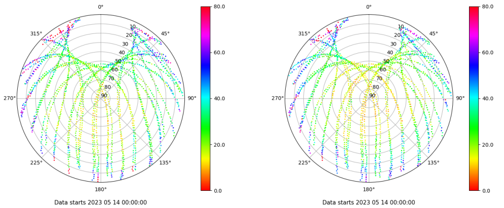
Skyplot for station ZFRA. Parameter M1C Data file ZFRA00ESP_R_2023134.xtr Skyplot for station ZFRA. Parameter M2P Data file ZFRA00ESP_R_2023134.xtr
